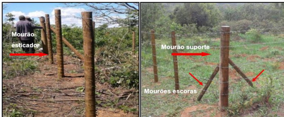
Figura 21 – Fotos Ilustrativas do modelo adotado para cercamento das nascentes Fonte: Localmaq (2017) - Município de Lassance, adaptado por SAMENCO (2019)
